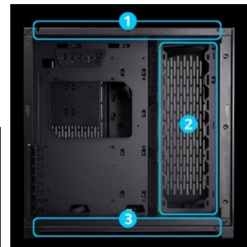
↑ラジエーター配置図
